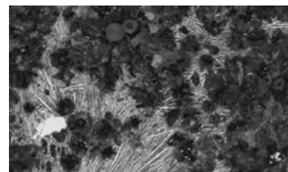
Carbonetos
